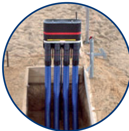
Mehrspartenhauseinführung im Bau
